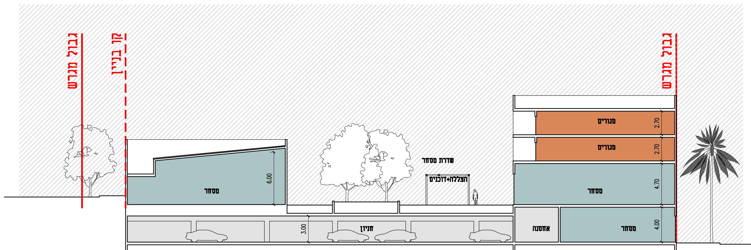
חתך 1-1
